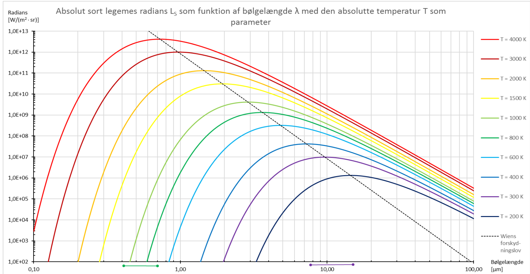
Figur 5: Kurveskarer, som viser radianse L_\lambda givet ved Ligning 5 for et absolut sort legeme som funktion af bølgelængden \lambda med den absolute temperatur T som parameter. Den stiplede sorte linje indikerer toppunktet for de enkelte temperaturkurver. Denne sammenhæng er kendt som Wiens forskydningslov.
