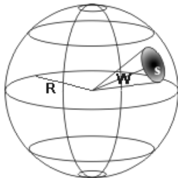
Figur 4: Illustration af en strålingsmåler med arealet S , som måler på et legeme, der befinder sig i kuglens midte. Afstanden mellem måleren og legemet er R .
