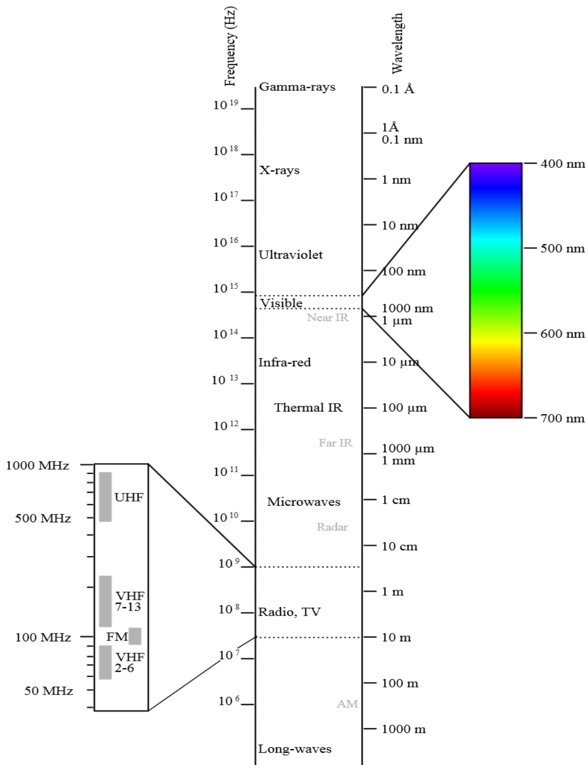
Figur 3: Frekvens- og bølglængdeinterval for den praktiske anvendelse af EM-bølger. I dette kompendie behandles bølglængder i området fra nogle μm til flere gange 10 μm (området benævnt "Infra-red").
